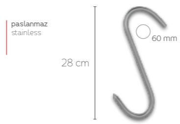
81053 Butcher's PKG S Çengel Paslanmaz S Hook 10 mm
